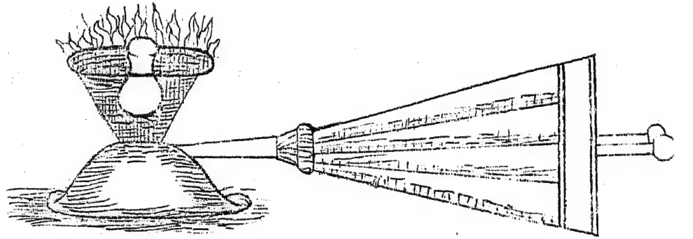
कोष्ठीयन्त्रम् १८
